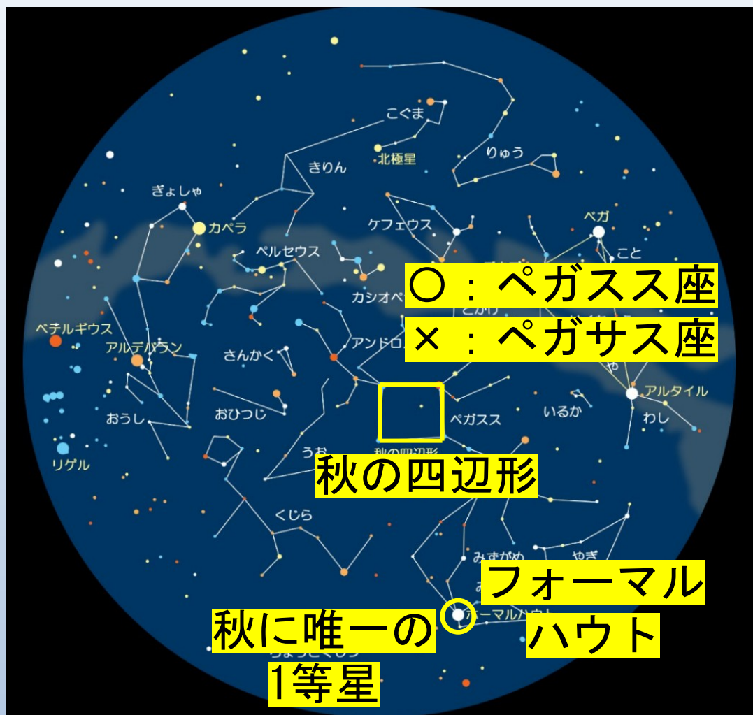
秋の星座
